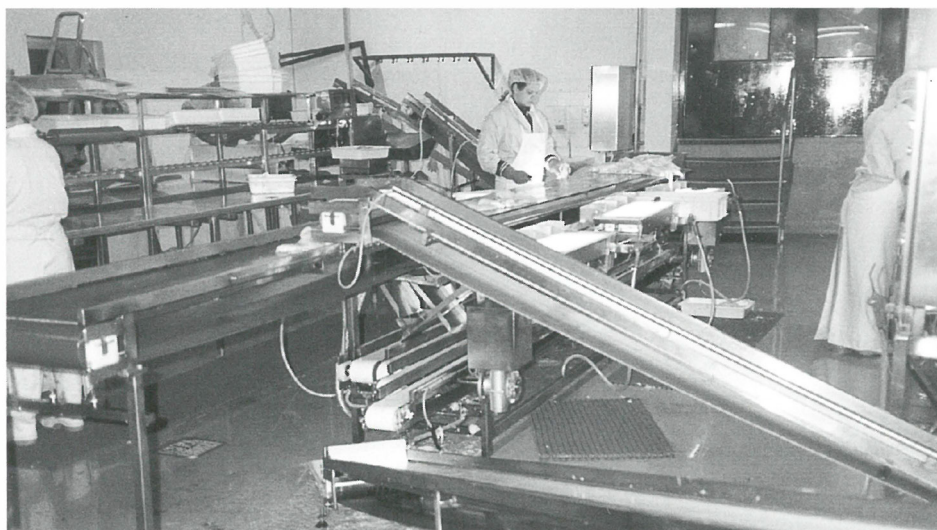
Flæðilína hjá Sjávarréttum hf. í Keflavík, tekin í notkun 1992.
