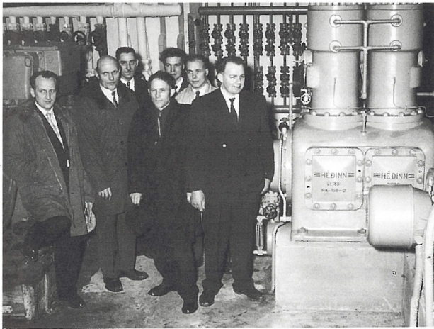
Fyrsta íslenska frystivél, smíðuð af Héðni, var sett upp í Heimaskaga árið 1950 og er myndin tekin þegar vélin var gangsett í fyrsta skiptið. Sveinn Guðmundsson í Héðni er lengst til vinstri, Bjarni Guðjónsson, vélæftirlitsmaður SH, er þriðji frá vinstri.
